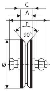
Y-profil
