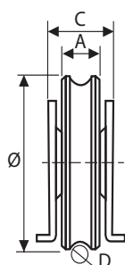
U-profil
