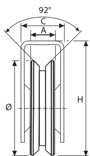
Y-profil
