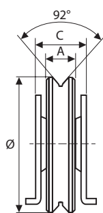
Y-profil
